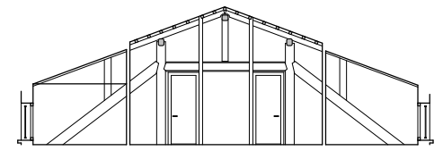
SEZIONE SCHEMATICA CAPRIATA A-A
